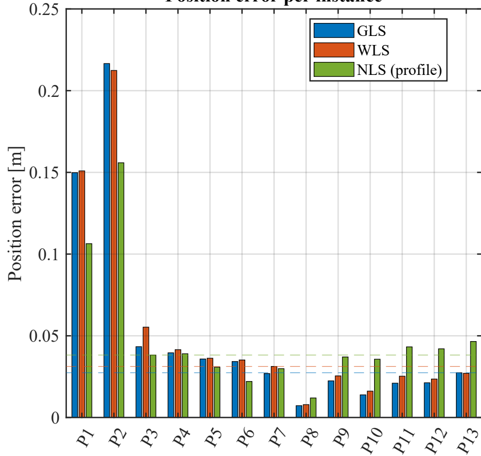
Position error per instance
