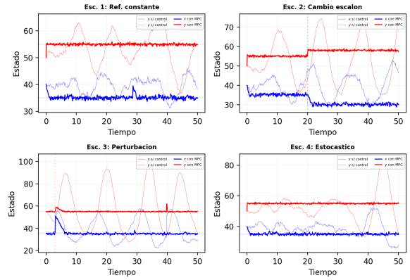
Figura 2: Comparativa por escenario (sin control en transparencia, con MPC en trazo intenso). Cada panel muestra un escenario de la Tabla 1. Las figuras individuales comparativa_escenario1-4.png amplían cada caso.
