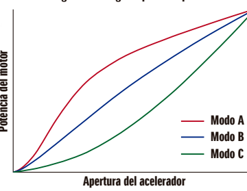
Imagen de entrega de potencia por modo
