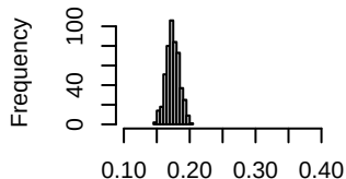
delta=1
