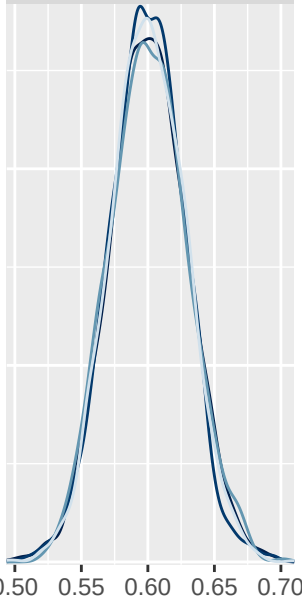
b_BMI
