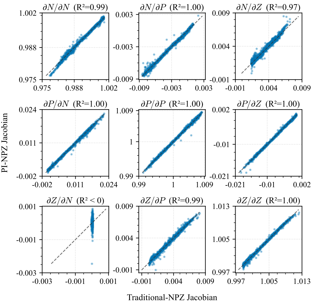
(a) Traditional-NPZ vs PI-NPZ
