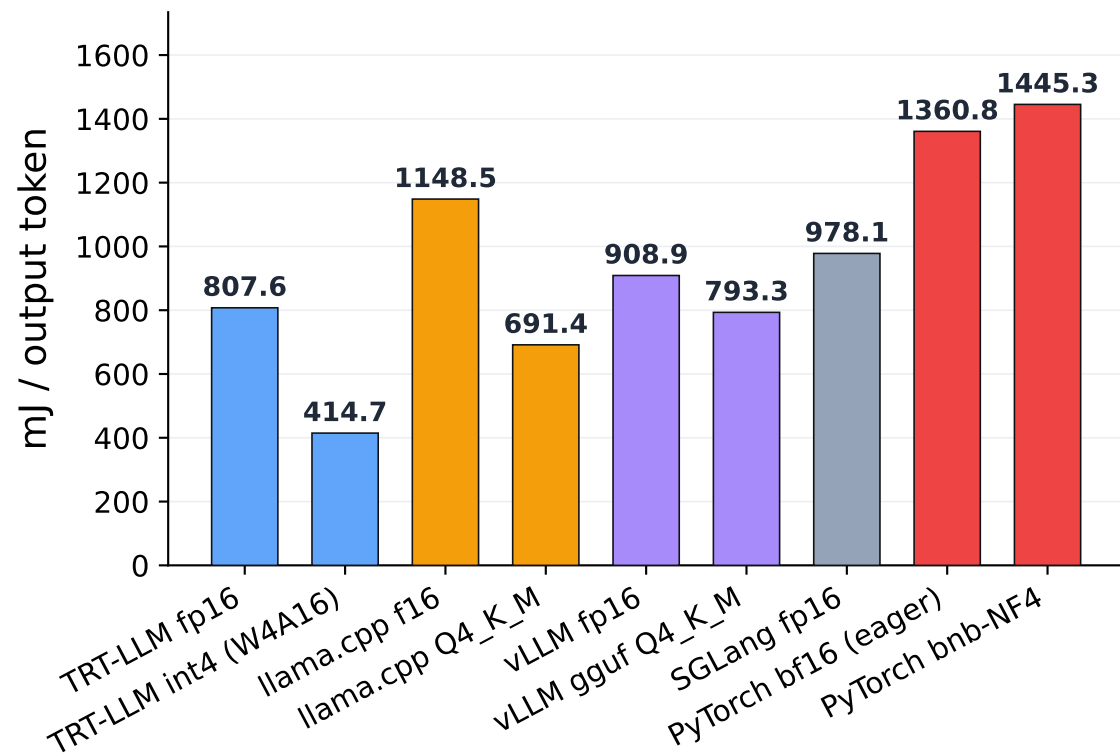
(d) Decode energy / output token
