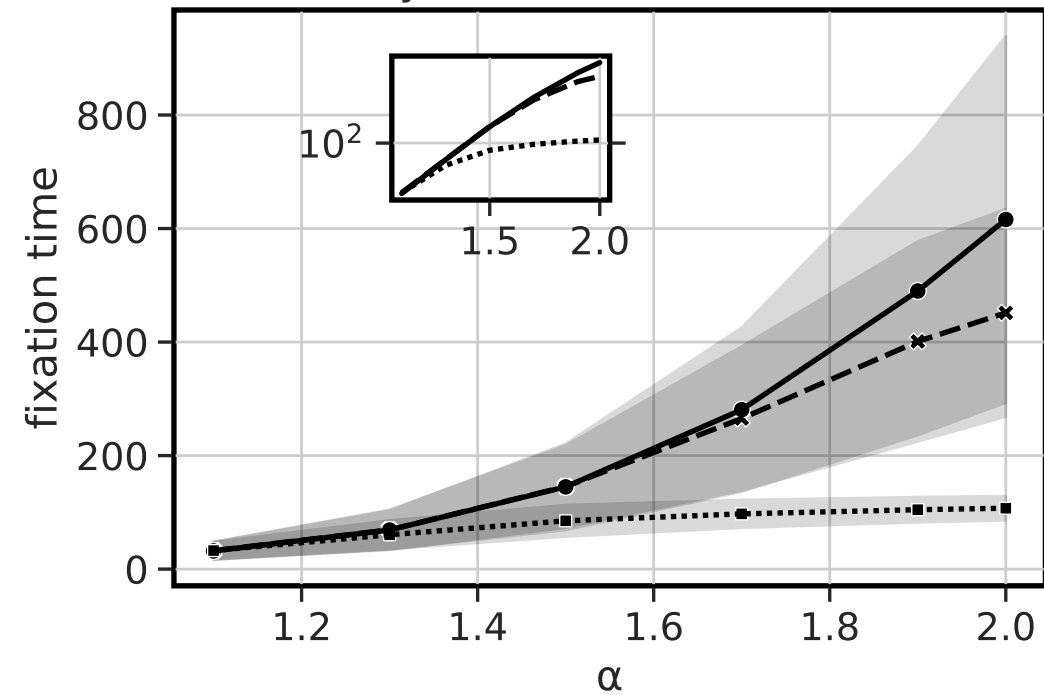
e) fecundity selection (N=1000)
