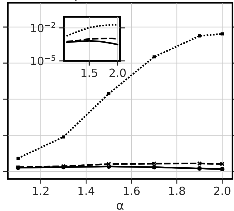
e) fecundity selection (N=1156)
