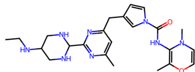
Rank 9 QED 0.52 | SA 4.10 Pred. KIBA 11.50
