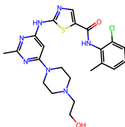
Rank 13 QED 0.47 | SA 2.65 Pred. KIBA 11.27
