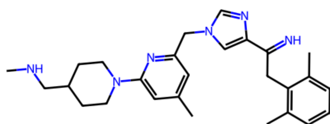
Rank 16 QED 0.51 | SA 3.08 Pred. KIBA 10.93
