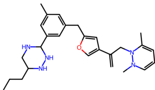
Rank 5 QED 0.55 | SA 4.73 Pred. KIBA 11.60
