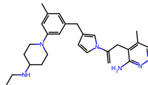
Rank 7 QED 0.54 | SA 3.34 Pred. KIBA 11.65
