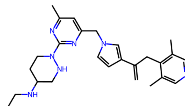
Rank 3 QED 0.55 | SA 4.06 Pred. KIBA 11.78
