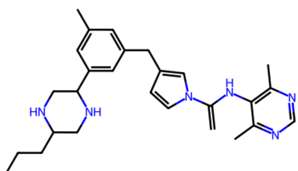
Rank 12 QED 0.47 | SA 4.24 Pred. KIBA 10.95
