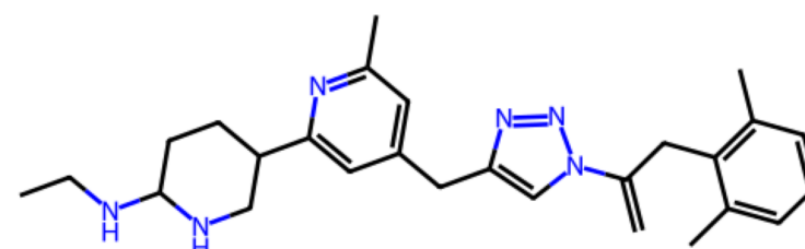
Rank 6 QED 0.54 | SA 4.22 Pred. KIBA 11.86
