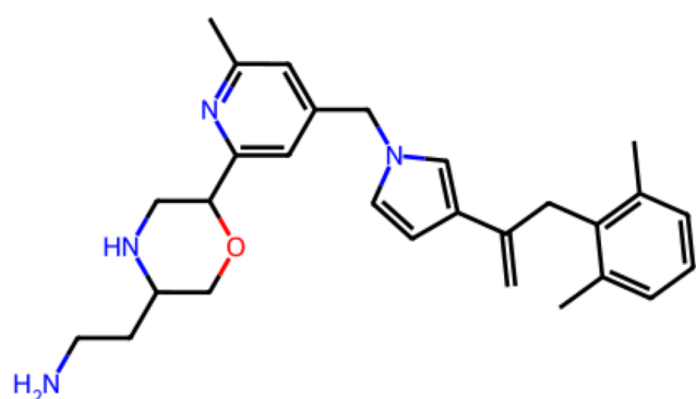
Rank 8 QED 0.54 | SA 4.12 Pred. KIBA 11.04
