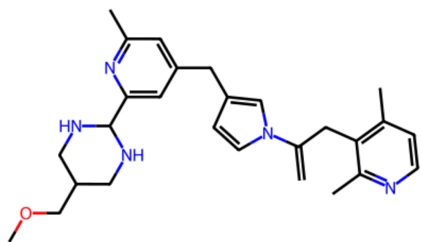
Rank 4 QED 0.55 | SA 3.74 Pred. KIBA 11.06
