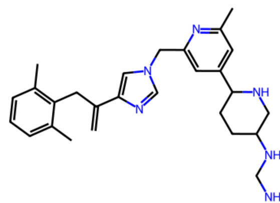
Rank 18 QED 0.46 | SA 4.15 Pred. KIBA 11.18
