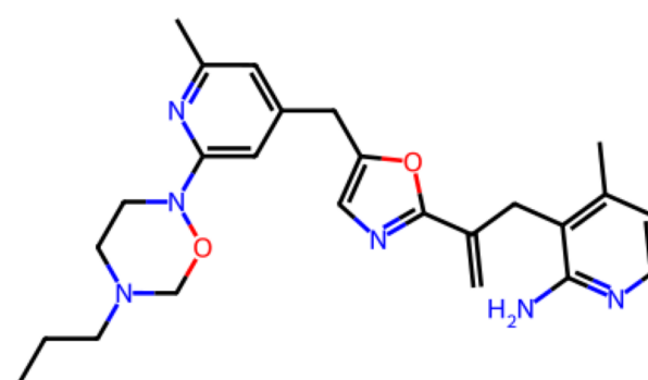
Rank 2 QED 0.55 | SA 3.71 Pred. KIBA 10.60
