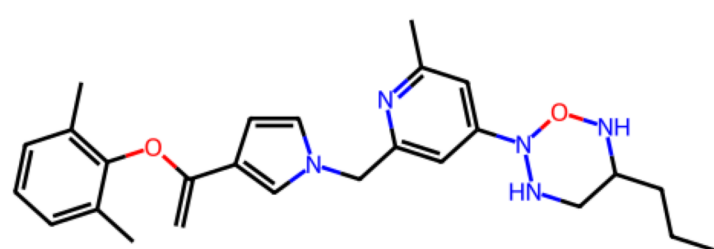
Rank 17 QED 0.48 | SA 4.15 Pred. KIBA 11.40
