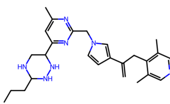
Rank 10 QED 0.49 | SA 4.51 Pred. KIBA 10.88
