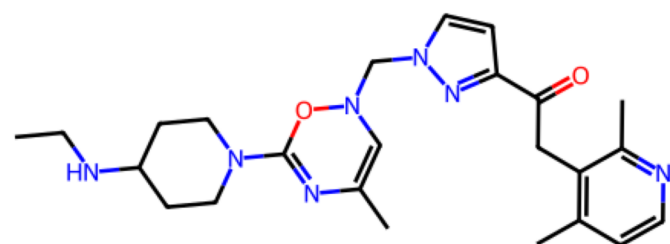
Rank 1 QED 0.65 | SA 3.60 Pred. KIBA 11.73
