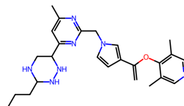
Rank 19 QED 0.46 | SA 4.49 Pred. KIBA 11.52
