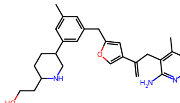
Rank 14 QED 0.46 | SA 4.04 Pred. KIBA 11.26
