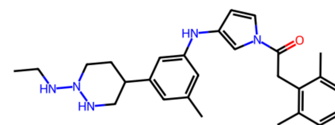
Rank 11 QED 0.48 | SA 3.82 Pred. KIBA 11.01
