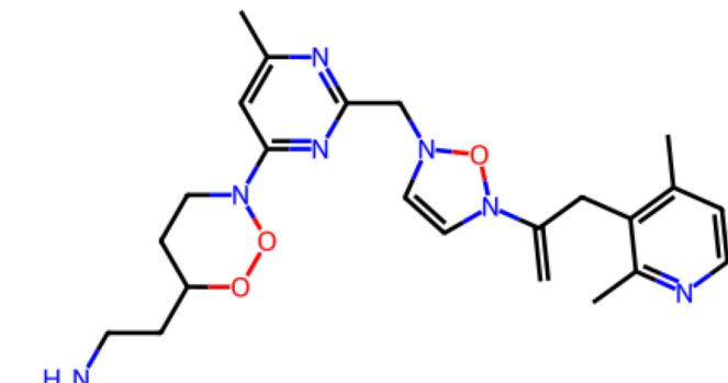
Rank 15 QED 0.60 | SA 4.71 Pred. KIBA 11.14
