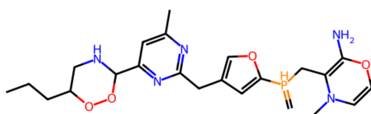
Rank 20 QED 0.44 | SA 5.50 Pred. KIBA 11.28
