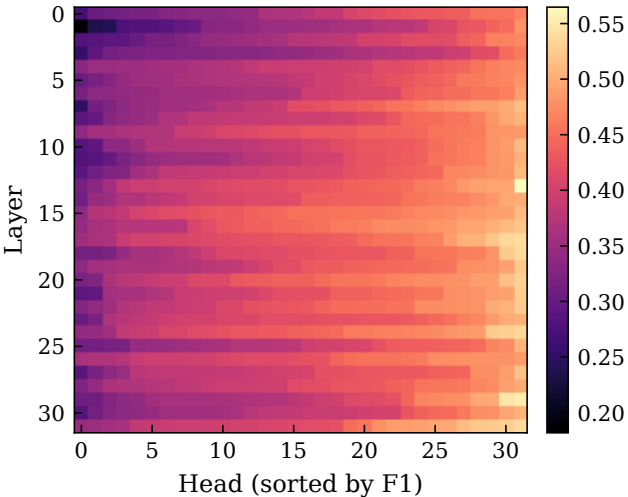
nfix / llama-3.1-8b
