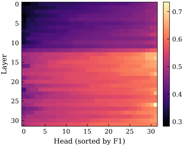
pond / llama-3.1-8b
