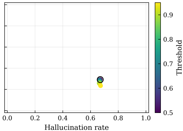
mistral-7b
