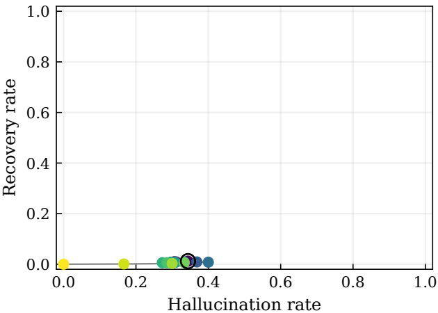
llama-3.1-8b
