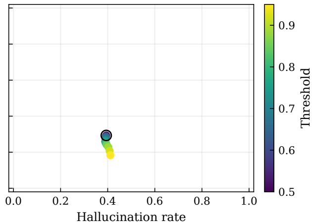
mistral-7b
