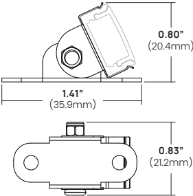
Pivot Clip
