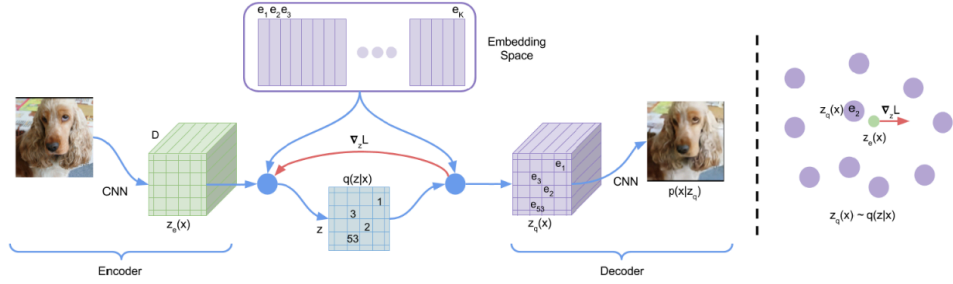
Figura 2 — A la izquierda, el pipeline de VQ-VAE. A la derecha, una representación del espacio de embedding
