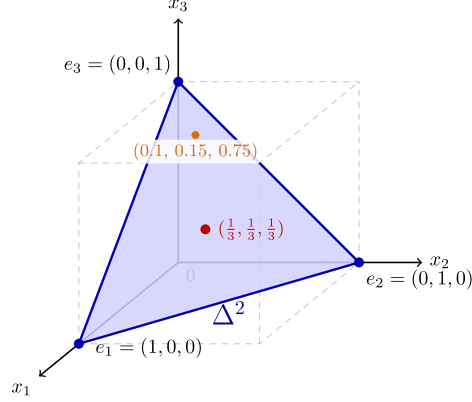
Figura 3 — Gráfico del simplex \Delta^2 .
