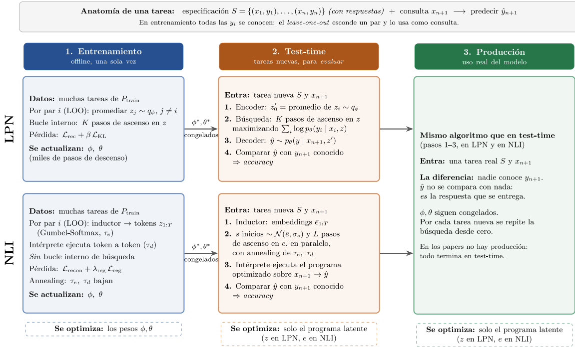
Figura 4 — Relación entre el funcionamiento de entrenamiento y producción de LPN y NLI
