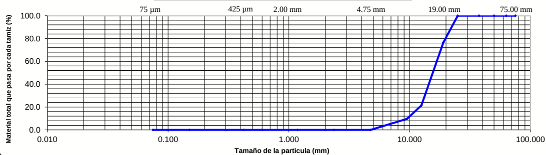
CURVA GRANULOMETRICA
