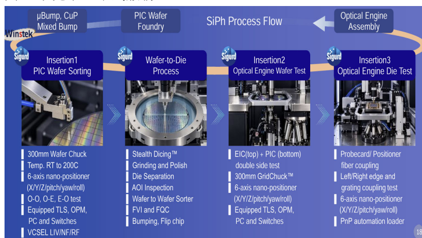
圖三.矽光子一站式服務
