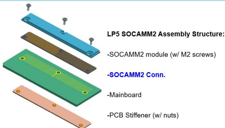
圖表 8：LPDDR5 SOCAMM2 連接器
