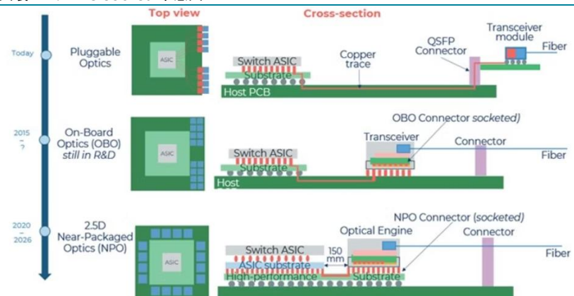
圖表 11：NPO socket 示意圖
