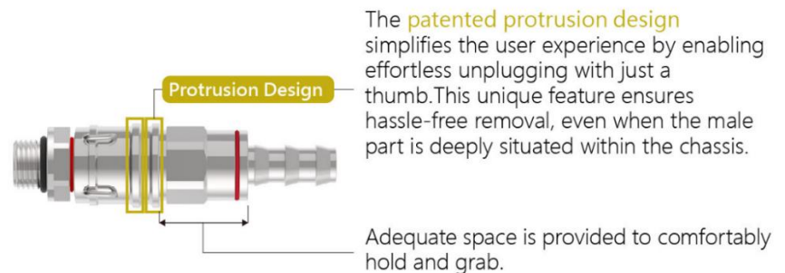
圖表 10：嘉澤 UQD 專利設計
