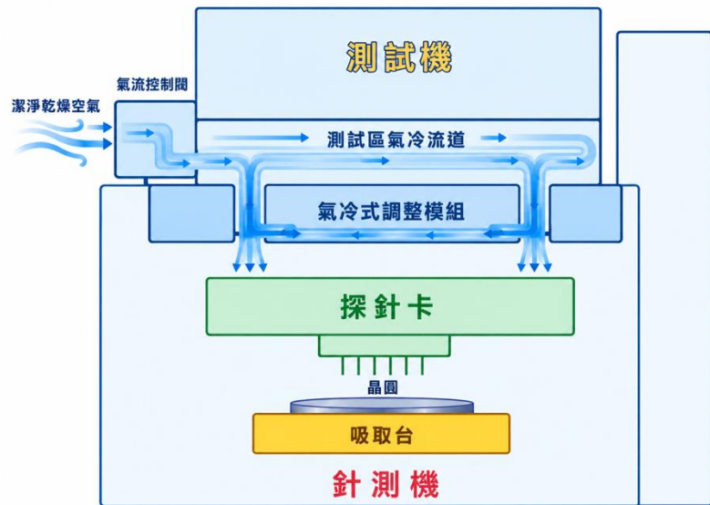
圖表 2: 漢測熱管理系統
