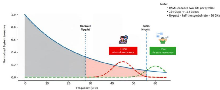
圖五、NV Rubin 精度要求 \pm 2\text{mil}
