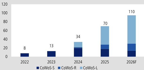
圖 62：CoWoS 產能擴充支應 AI 伺服器需求提高
