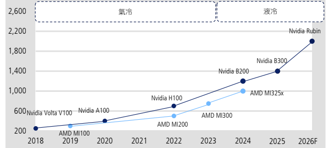
圖 65：GPU 散熱設計功耗(TDP)增長，將逐步帶動液冷散熱之需求
