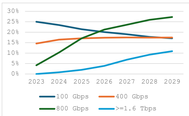
圖 3: 800G 交換器滲透率將超越 400G
