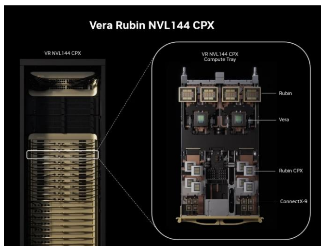
圖三、NV Vera Rubin NVL144 CPX
