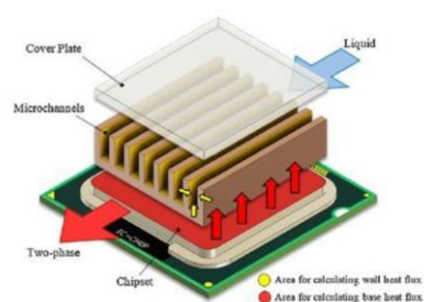
圖二、Micro channel lid 內部設計
