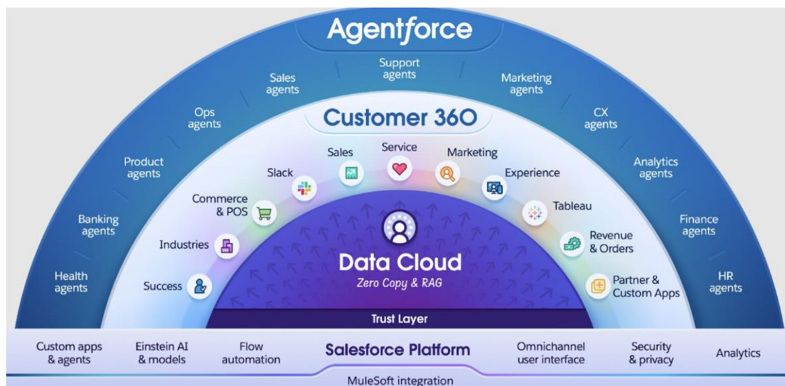
圖一、Salesforce 平台架構
