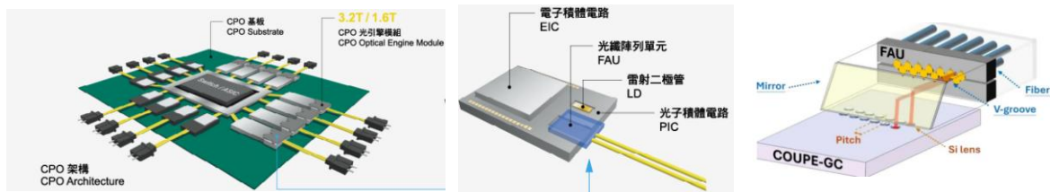
圖 4：CPO (共同封裝光學)需更高精度 FAU (左)(中)；COUPE 架構需要微稜鏡折射(右)
