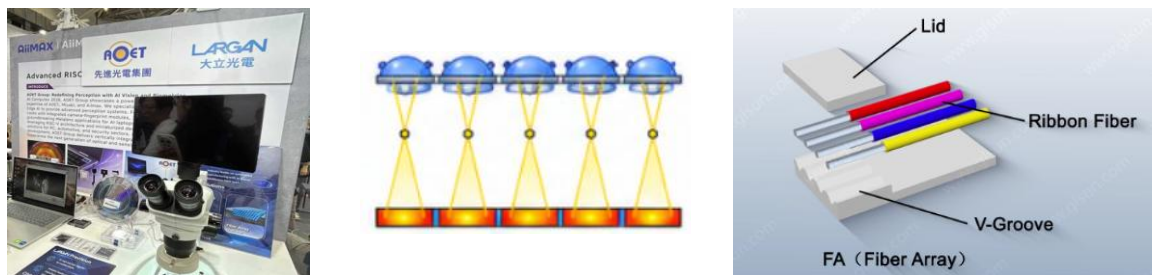
圖 3：大立光於 Computex 展出 FA、PMLA 及 V-Groove (左)；PMLA 可使目標面形成多點聚焦能量集中(中)；FA 利用 V-Groove 將多根裸光纖並排固定在基板上(右)
