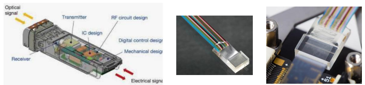
圖 5：插拔式光收發模組(Optical Transceiver)內部亦具 FAU(左)；FAU 功能是作為外部光纖與晶片之間的光學連接橋樑，將多路光纖以高精度固定並引導(中、右)
