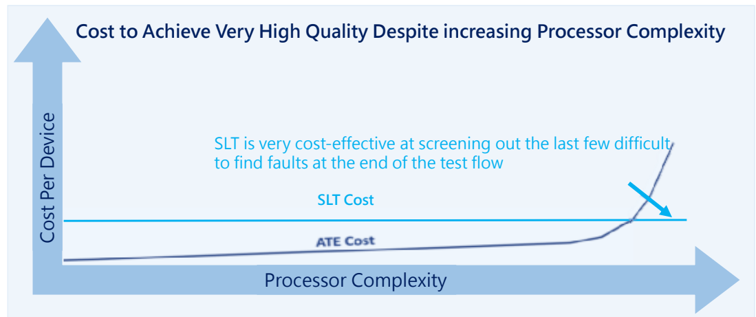
圖 16：隨晶片複雜度提升，SLT 能有效減少封裝後的測試成本
