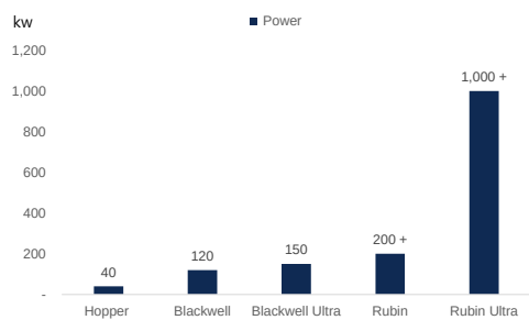
圖 10：Nvidia 機櫃瓦數未來將急遽提升
