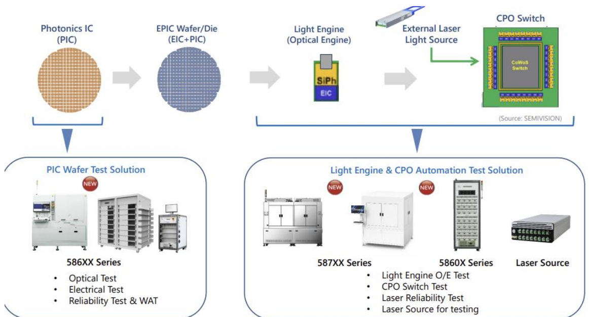
圖 3：致茂新通過驗致之 CPO Tester 主要用於 OSAT 端的 Die Level Test (圖右下)
