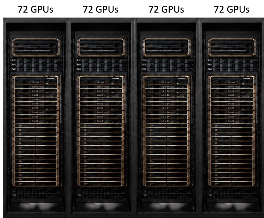
圖表 6：四櫃 Oberon 機架設計
