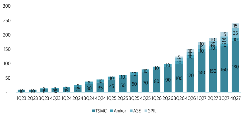
圖表 3：台積電 3D fabric 聯盟可用產能
