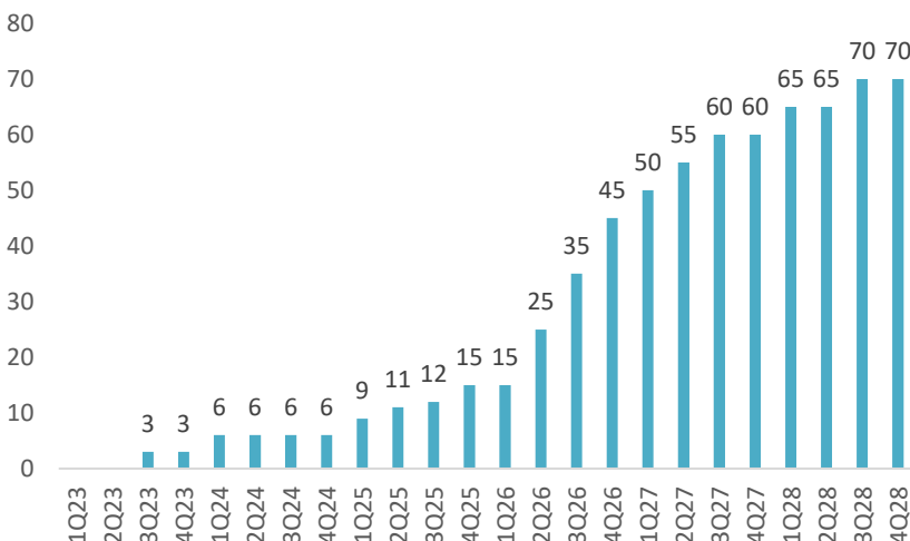
圖表 4：台積電 SoIC 產能預估
