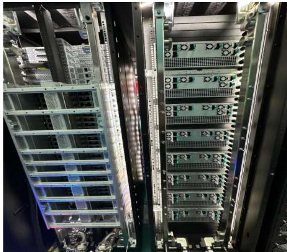
光寶液冷解決方案(背面)
