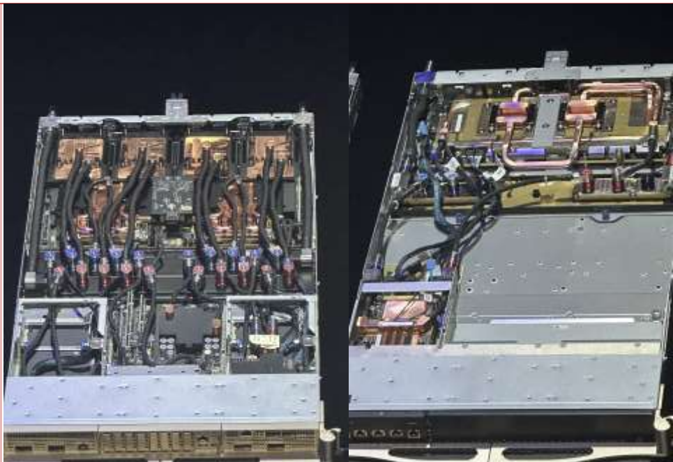
Cordelia架構 的Compute Tray(左)及 NVSwitch Tray(右)
