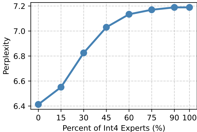
WikiText
