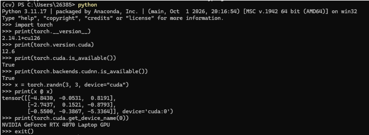
图4 PyTorch、CUDA、cuDNN 与 GPU 矩阵运算验证
