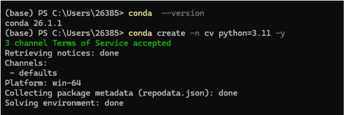
图1 conda 版本检查与 cv 环境创建
