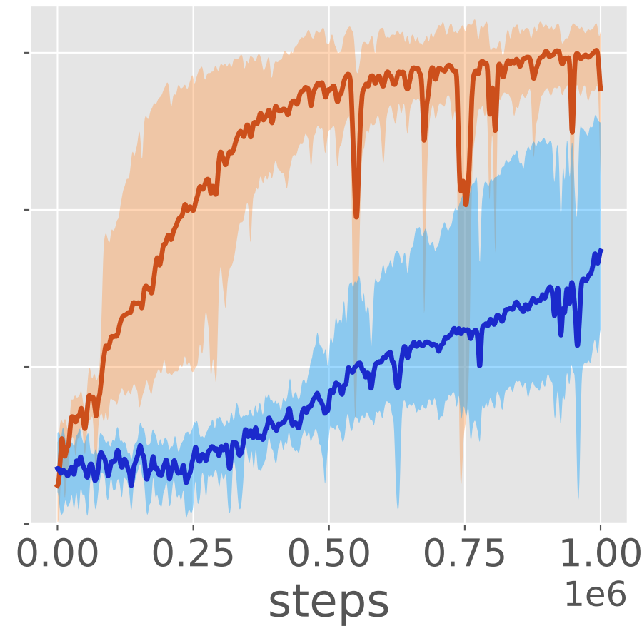
Ant
