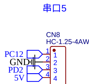
雷达接口
