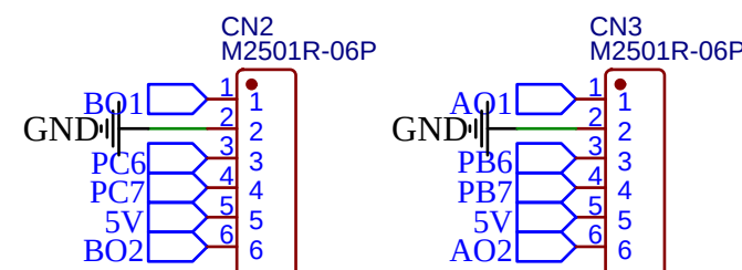
电机接口
