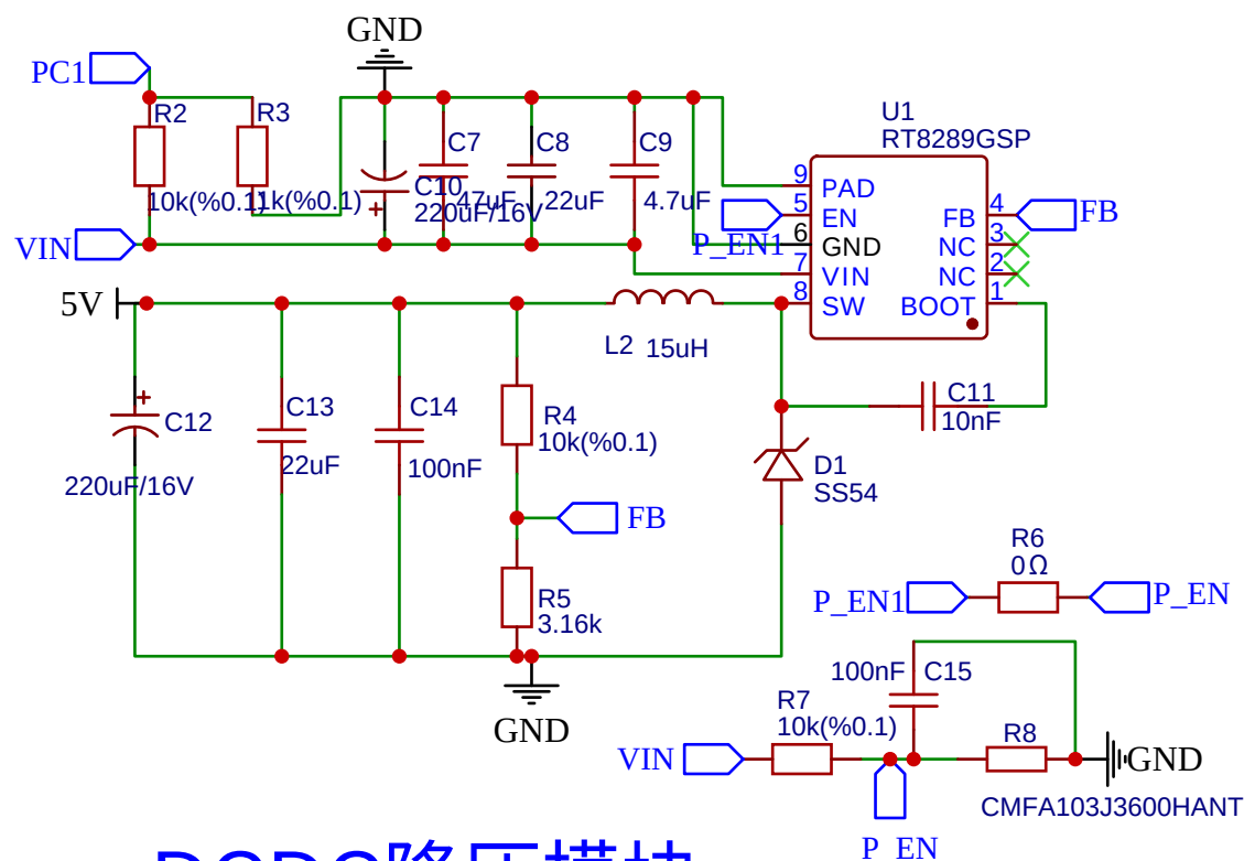
DCDC降压模块
