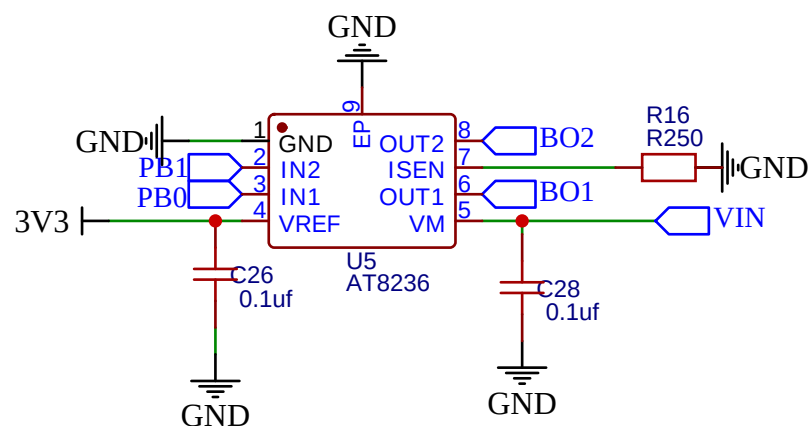
双电机驱动
