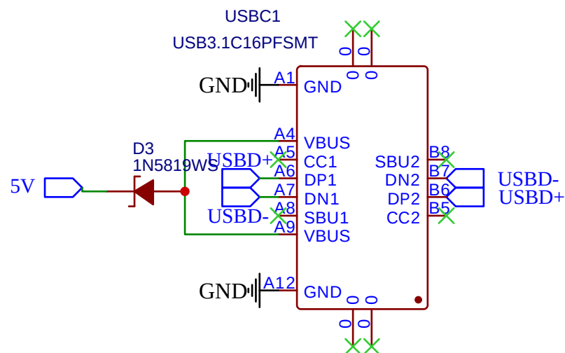
TYPE-C接口
