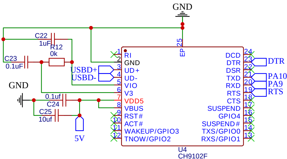
串口模块
