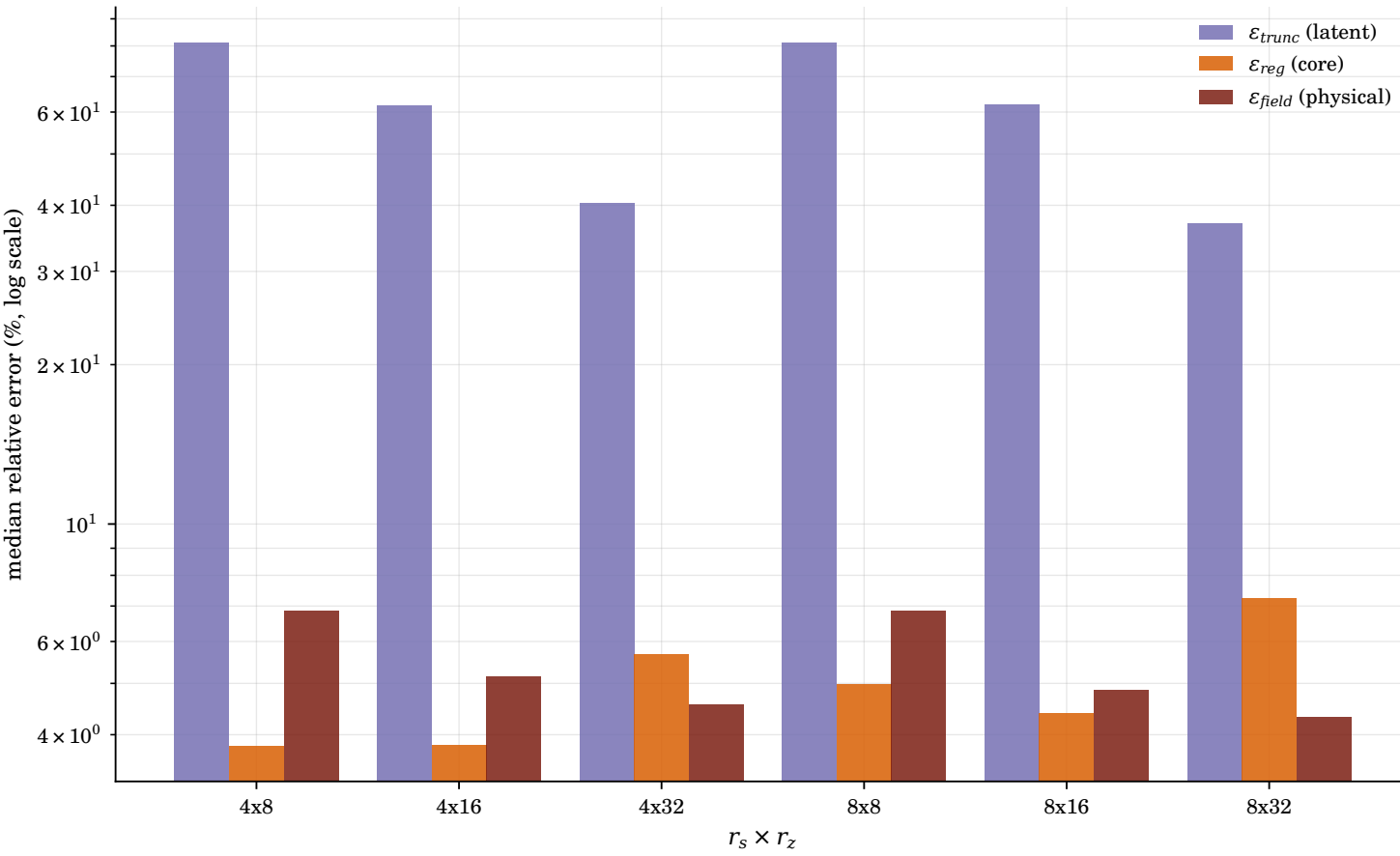
LLAE-Tucker
