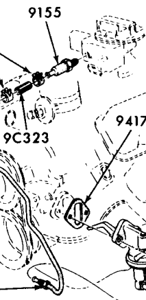
8 CYL. 302-2V, 351-2V, & 390-2V ENGINES
