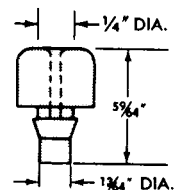
354860-S (CC-6)
