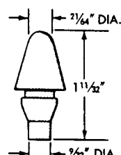
359933-S (CC-33)
