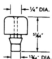
377781-S (CC-34)
