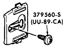
379560-S (UU-89-CA) DIOZ-6520818-A LB
