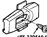
USE 379560-S (UU-89-CA) C9AZ-6220818-A W
