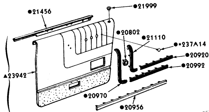
FRONT DOOR
