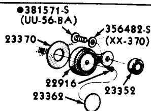
FRONT DOOR
