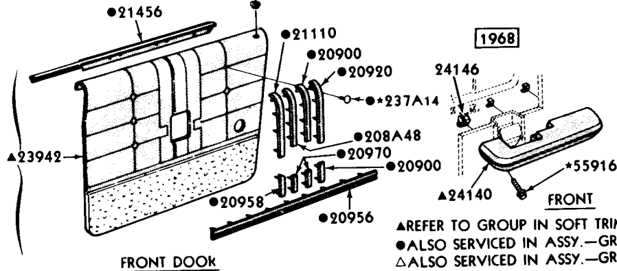
FRONT DOOR
