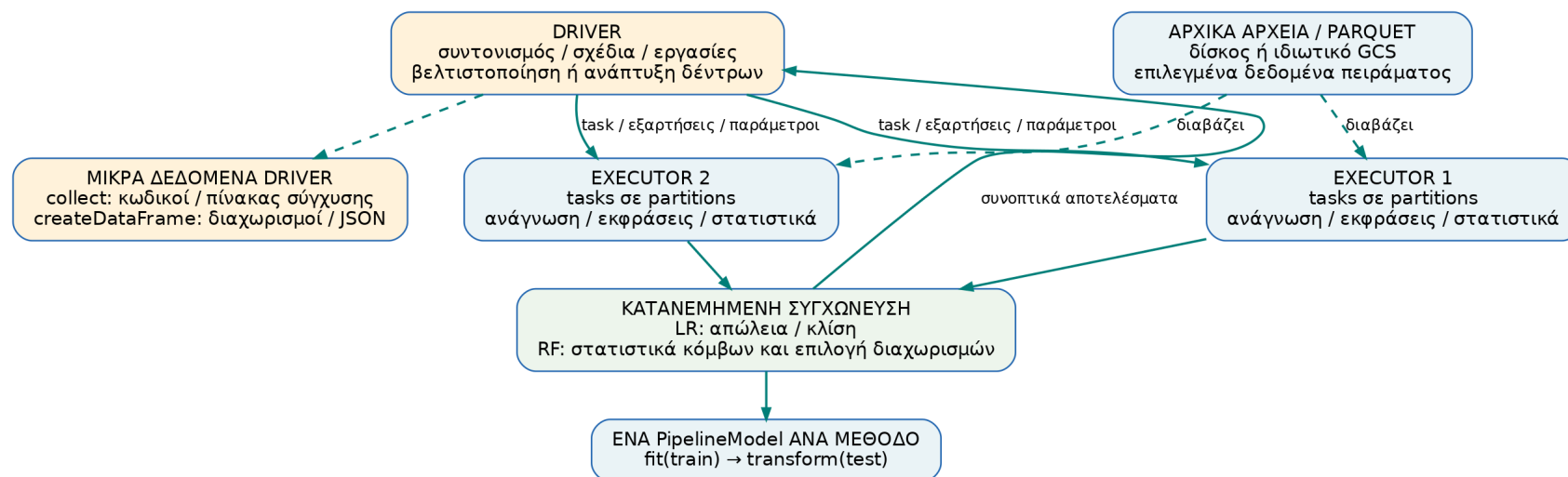
Σχήμα 3. Ανάγνωση, συντονισμός και μικρά αποτελέσματα. Πηγή: ο κώδικας εφαρμογής και οι Spark ML αλγόριθμοι.
