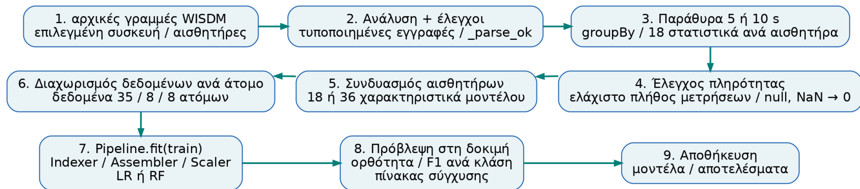
Σχήμα 1. Ροή δεδομένων και μοντέλων. Πηγή: ingest.py , features.py , model.py , pipeline.py .
