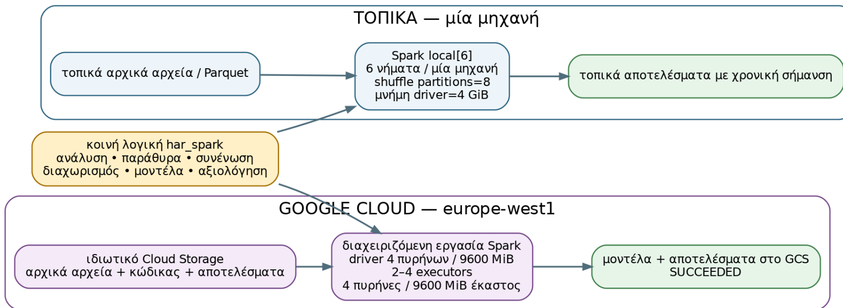
Σχήμα 6. Ρυθμίσεις τοπικής και καταγεγραμμένης cloud εκτέλεσης. Πηγή: YAML και cloud/deployment.md.
