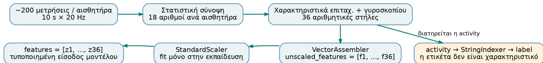
Σχήμα 5. Aggregation, σύντηξη, VectorAssembler και train-fit StandardScaler. Πηγή: features.py και model.py.
