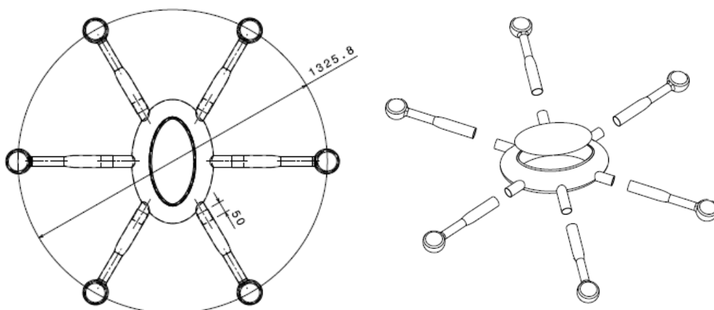
Figura 6. Planta y vista isométrica del RPA CÓNDOR
