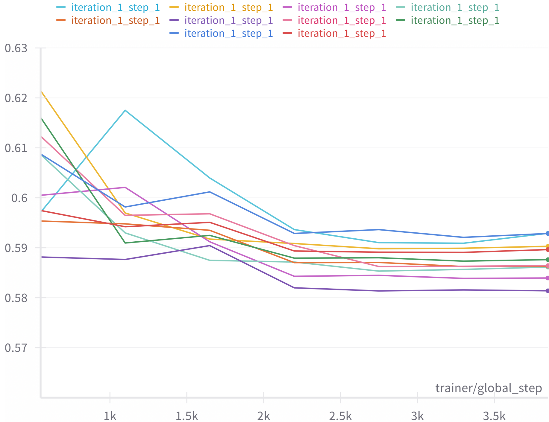
val_loss
