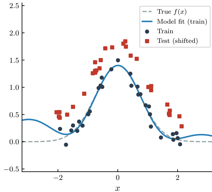
Domain Shift
