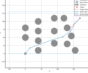
F1 (TD): 0.02, F2 (Len): 210.6, F3 (Und): 1.00, F4 (# Seg): 7
