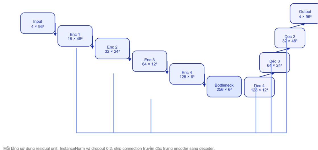
Hình 3. Kiến trúc khái niệm 3D U-Net theo cấu hình kênh của notebook v2.
