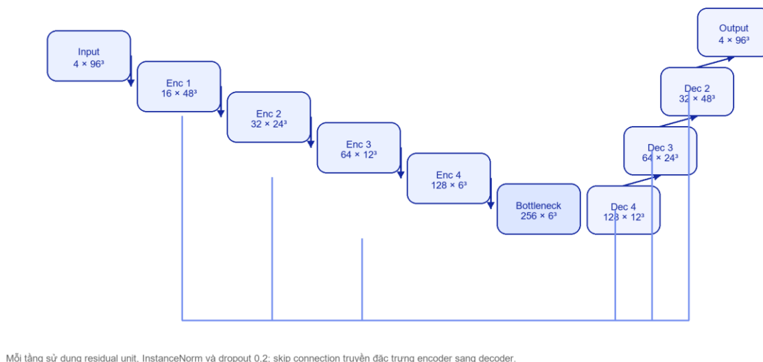
Hình 6. Kiến trúc khái niệm 3D U-Net theo cấu hình kênh của notebook v2.
