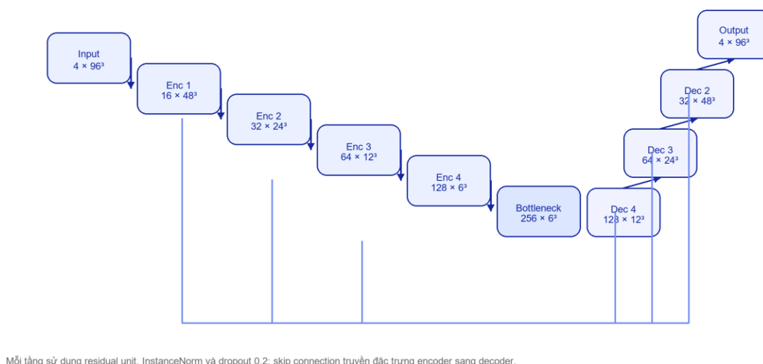
Hình 4. Kiến trúc khái niệm 3D U-Net theo cấu hình kênh của notebook v1.
