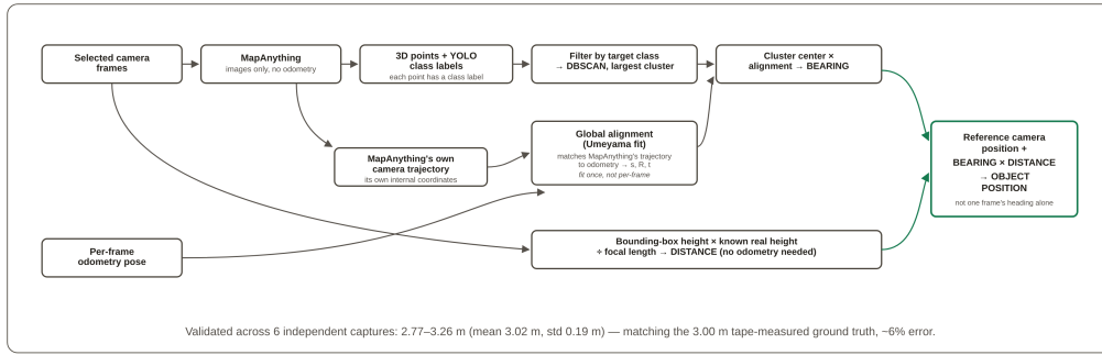
Hình 2: Pipeline định vị đối tượng bằng hướng từ cụm điểm ngữ nghĩa MapAnything kết hợp khoảng cách đơn-ảnh.
