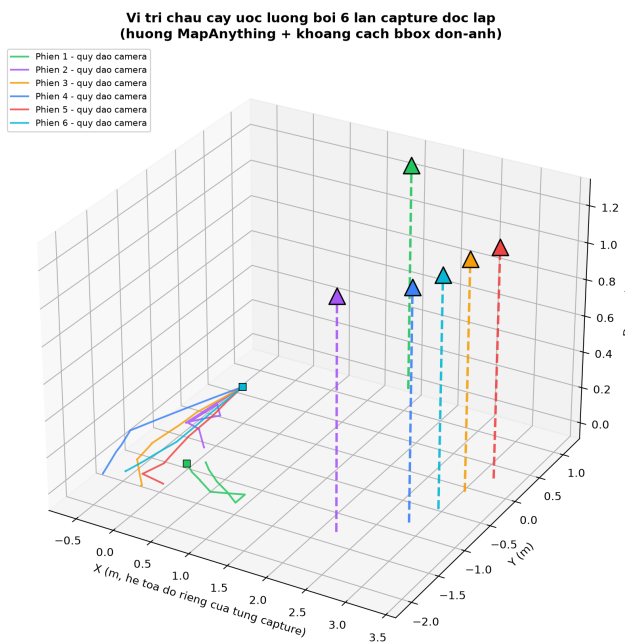
Hình 5: Quỹ đạo camera (đường liền, ô vuông = điểm xuất phát) và vị trí chậu cây ước lượng (tam giác + đường đứt, cao 1,25 m — chiều cao thật của cây) của sáu phiên chụp, mỗi phiên trong hệ toạ độ riêng gốc tại điểm xuất phát.
