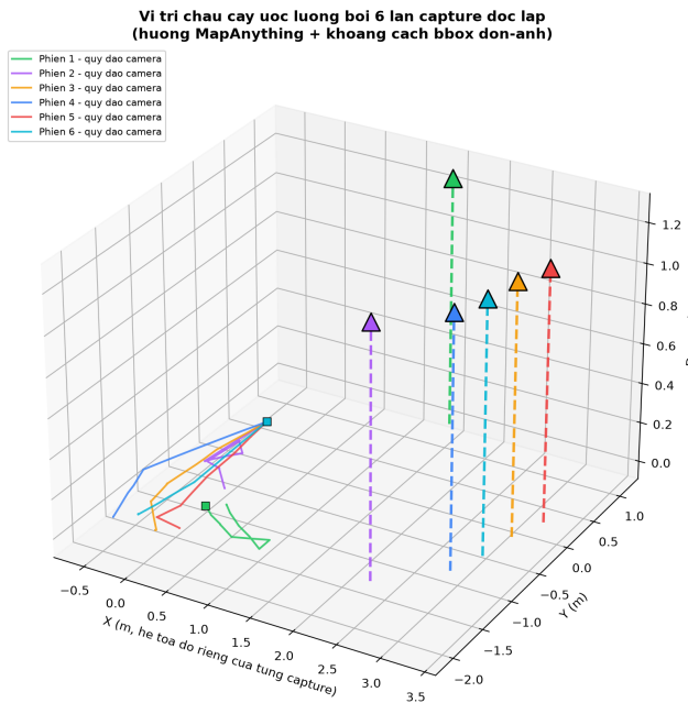
Hình 6: Quỹ đạo camera (đường liền, ô vuông = điểm xuất phát) và vị trí chậu cây ước lượng (tam giác + đường đứt, cao 1,25 m — chiều cao thật của cây) của sáu phiên chụp, mỗi phiên trong hệ tọa độ riêng gốc tại điểm xuất phát.
